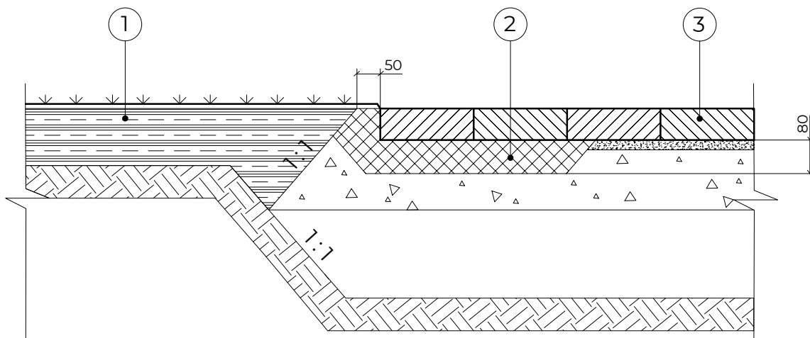
Илл. 1.3.2. ПРИМЫКАНИЕ МОЩЕНИЯ К ГАЗОНУ: 1 – ГАЗОН; 2 – РАСТВОР НА ОСНОВЕ ЦЕМЕНТНОГО, ТРАССОВО-ЦЕМЕНТНОГО ИЛИ ПОЛИМЕРНОГО ВЯЖУЩЕГО; 3 – МОЩЕНИЕ
