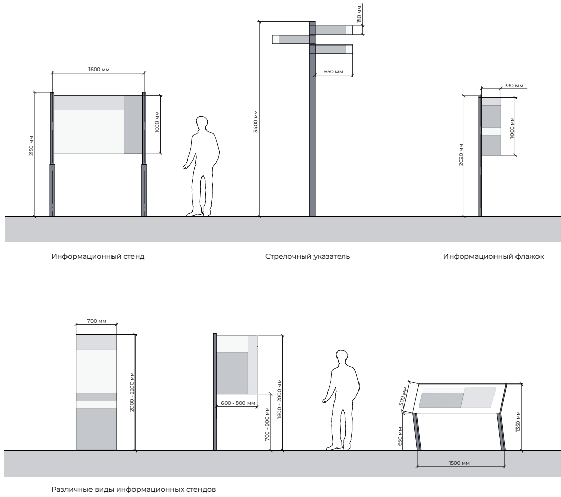
Илл. 5.7.4. ГАБАРИТЫ ОБОРУДОВАНИЯ ДЛЯ НАВИГАЦИИ
